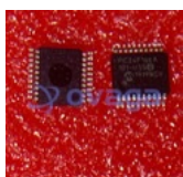
PIC24F16KA101-I/SS
